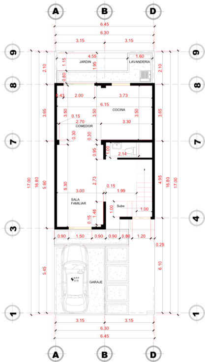
PLANTA ACOTADA CASA HABITACIONAL-VERONA 2 PRIMER NIVEL
